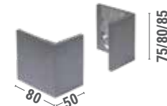
ANGOLARE A SOFFITTO ANGULAR CEILING MOUNTING
