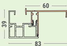
PROFILO CHIUSURA PER INCASSO OPTIONAL COVER FOR ENCASEMENT
