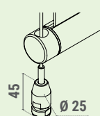
CILINDRO TENDICAVO CABLE TENSIONING UNIT
