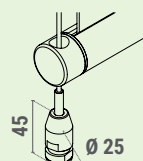
CILINDRO TENDICAVO CABLE TENSIONING UNIT
